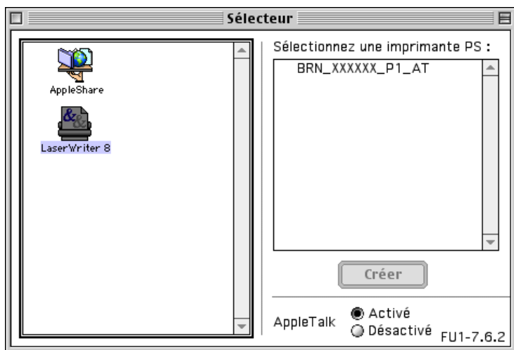
Figure 2 Sélecteur Macintosh
