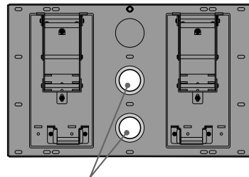
Foro per il passaggio dei cavi (uno di due)
