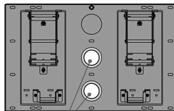
Hål för kabeldragning (ett av två)
