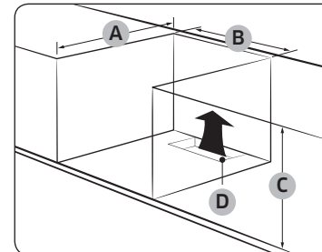
Gootstenkast (mm)
