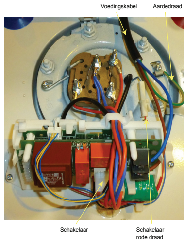
Verticaal wandmodel
