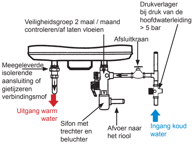
Aansluitschema (voorbeeld van een verticaal wandmodel)
