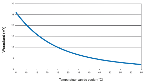
Verhouding tussen weerstand van de thermostaatvoeler en de temperatuur
