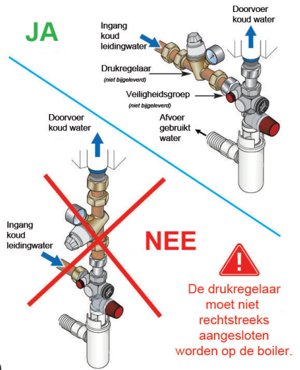
Aansluitschema (voorbeeld van een verticaal wandmodel)
