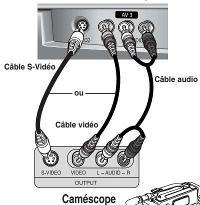
Panneau latéral du téléviseur (HC-P4252W)
