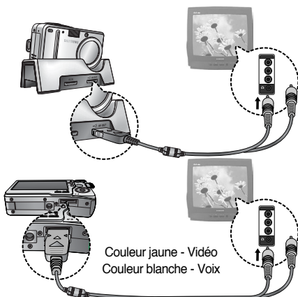
[Utilisation du câble AV avec le support]
