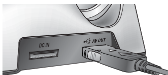
[Utilisation du câble USB avec le support]
