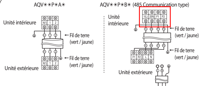
Unité extérieure
