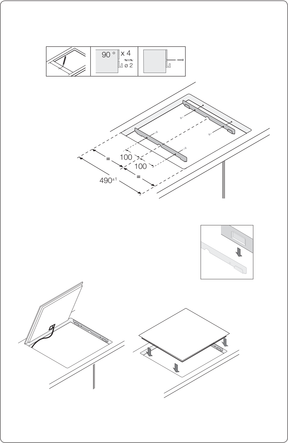
Installation de la table de cuisson _15
