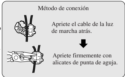
Cable de la luz de marcha atrás.
