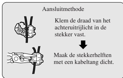
Draad van achteruitrijlicht.
