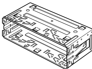
Supporto
