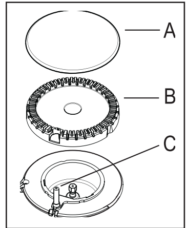
A - Chapeau du brûleur B - Coronne du brûleur C - Bougie d'allumage
