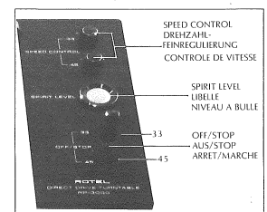
Figure 8. Control Panel Abbildung 8. Bedienungs-tafel Figure 8. Panneau de contrôle
