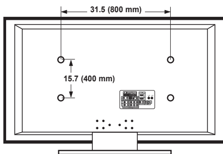
VUE ARRIÈRE
