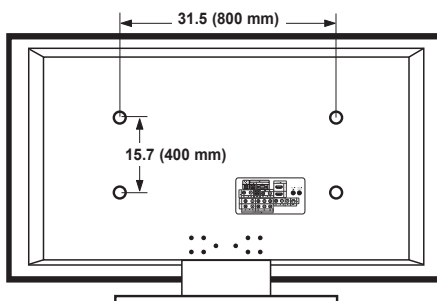
VISTA POSTERIOR
