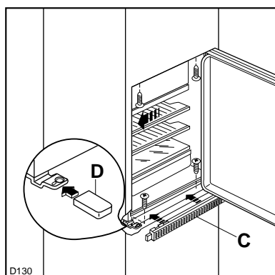
Fig. 4 Ouvrez la porte et appuyez l'appareil contre le meuble de cuisine, du côté opposé aux charnières. Fixez l'appareil à l'aide de 4 vis. Appliquez la grille d'aération (C) et le couvre-charnière (D).
