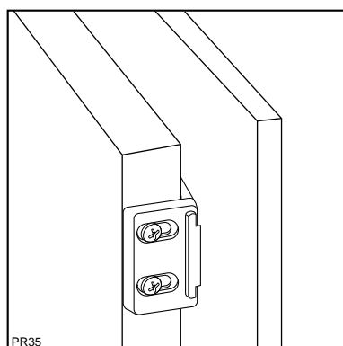
Fig. 9 Enlevez les équerres et faire des trous de Ø 2 mm. Remettez les équerres au-dessus des guides et vissez le tout avec les vis fournies en accessoires (3,5x16 mm). Pour aligner la porte du meuble, si cela est nécessaire, recourez
