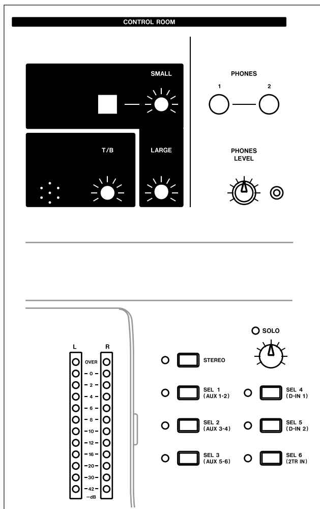
Figure 4.7: Commandes d'écoute et d'affichage de niveau
