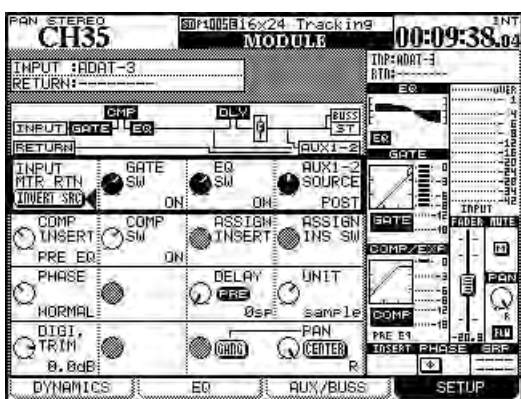
Figure 5.14: Ecran Setup de module de voie
