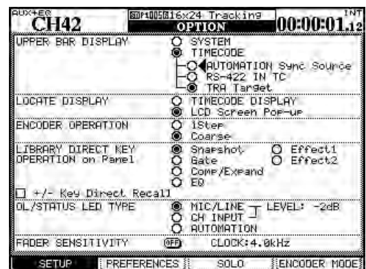
Figure 2.38: L'écran option SETUP
