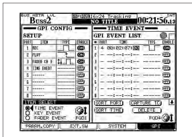
Figure 2.44: Ecran de réglage de GPI
