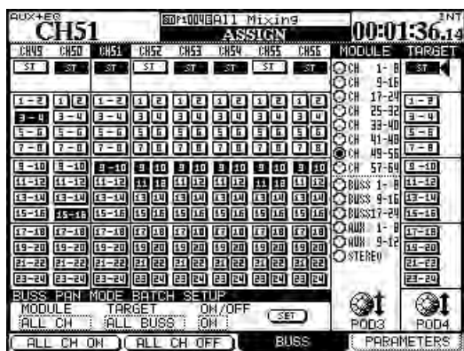
Figure 4.5: Ecran d'affectation de bus (bus couplés)
