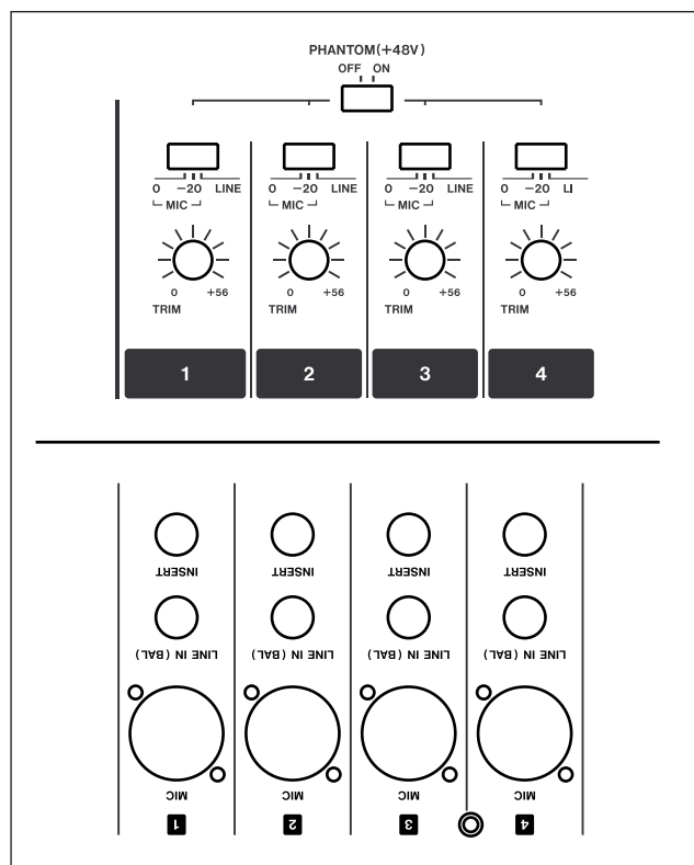
Figure 3.2: Entrées et commandes analogiques de voie
