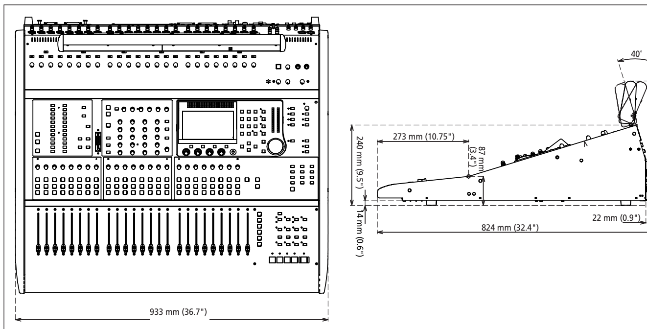
Figure 9.1: Dessin avec cotes (incluant le bandeau de vu-mètres MU-1000 optionnel)
