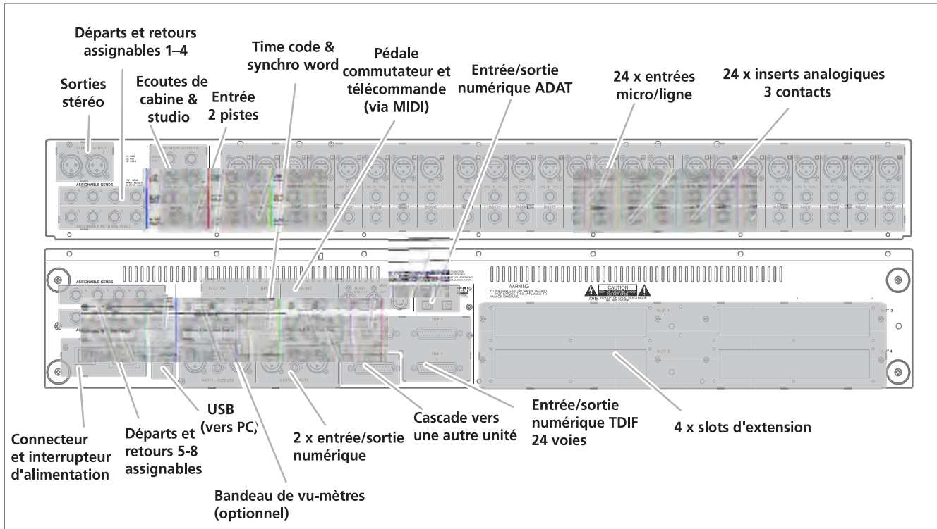
Figure 3.1: Organisation de la face arrière
