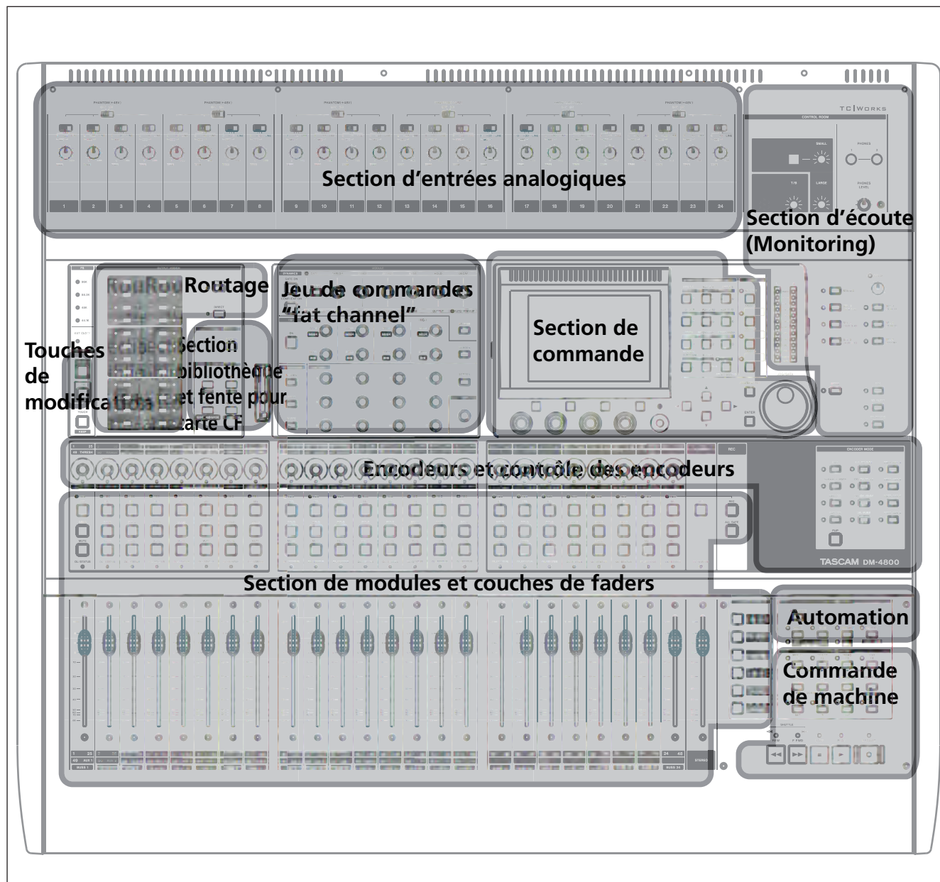
Figure 1.2: Survol de la DM-4800
