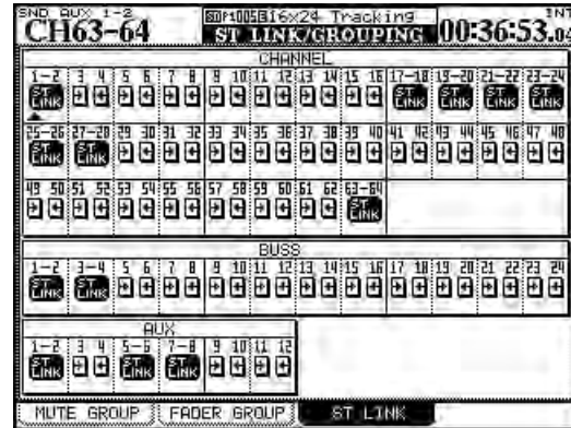
Figure 5.20: Ecran de couplage stéréo
