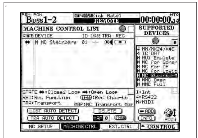
Figure 8.8: Configuration de commande de machine pour le contrôle du transport d'une station de travail audio numérique
