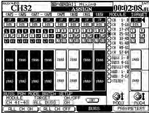
Figure 4.6: Ecran d'affectation des canaux surround
