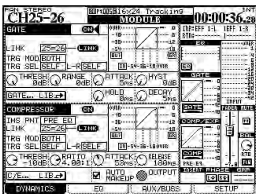
Figure 5.7: Ecran de processeur dynamique couplé (voies 1 à 48)
