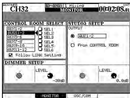
Figure 4.8: Ecran des paramètres d'écoute (Monitor)
