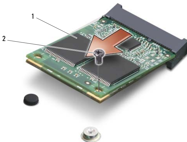
1 Carte FCM 2 vis M2 x 3 mm
