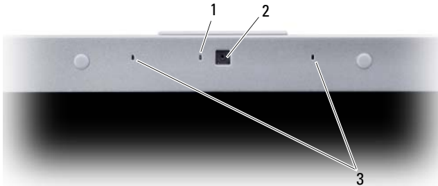
1 témoin de caméra 2 caméra 3 microphones numériques (2)
