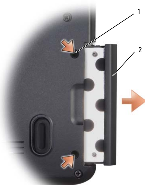
1 vis (2) 2 disque dur
