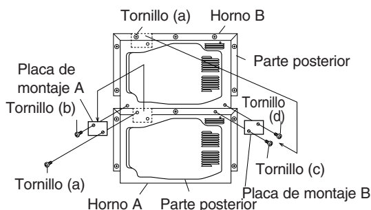
Figura A. Cómo instalar dos hornos
