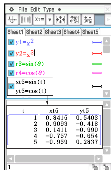
ParamType : table numérique ( t, xt, yt )
