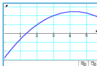
Graphe de régression quadratique
