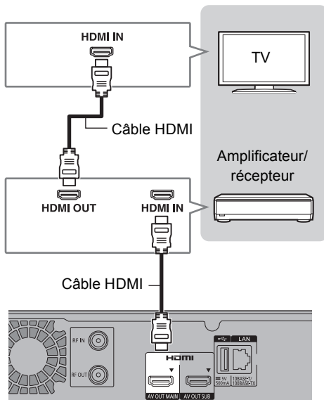
Décodeur TV (STB) ou équipement vidéo
