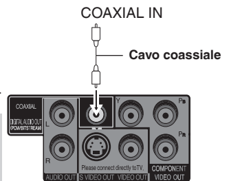
Parte posteriore dell'apparecchio
