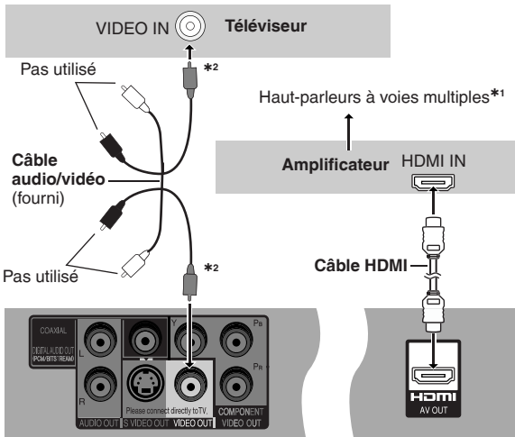
Panneau arrière de l'appareil
