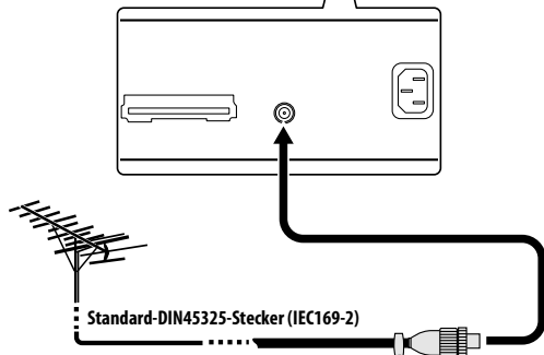
75-Ohm-Koaxialkabel (rund) (im Fachhandel erhältlich)
