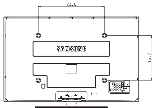
VISTA POSTERIOR
