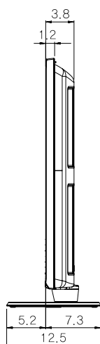
VUE LATÉRALE
