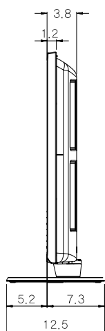
VISTA LATERAL
