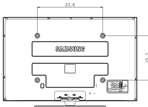
VUE ARRIÈRE
