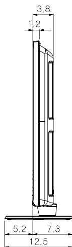
VISTA LATERAL
