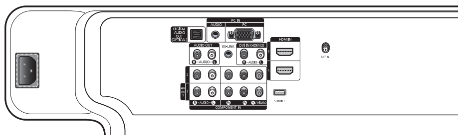
DIMENSION DU PANNEAU DE PRISES 3.7" H x 7.2" W
