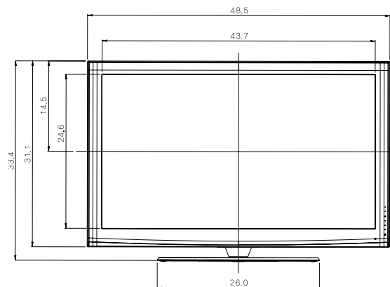
VUE AVANT
