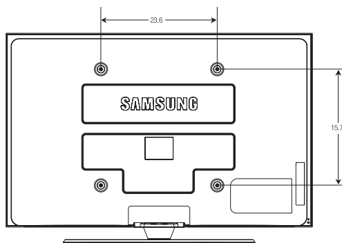
VUE ARRIÈRE
