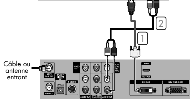
Décodeur pour télévision numérique (DTV)
