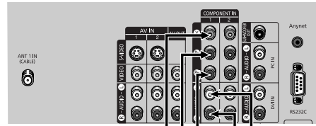
Panneau arrière du téléviseur
