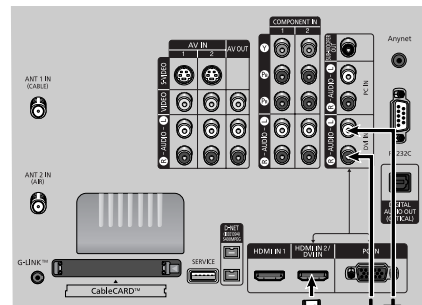
Panneau arrière du téléviseur
