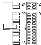
Connecteur d'alimentation principal (20+4 broches)
