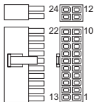
Conector principal de alimentación (20+4 pines)
