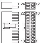
Главный разъем питания (20+4 контакта)
