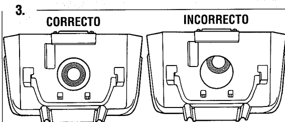
Diagrama 3 Asegúrese que la apertura de la bolsa esté alineada correctamente con la apertura en la conexión de la manguera.
