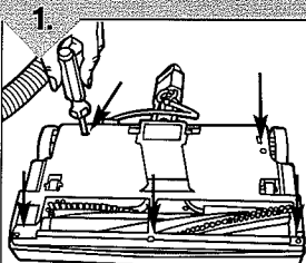
Diagrama 1 Para quitar la protección de la boquilla: voltee la boquilla eléctrica. Quite los cinco (5) tornillos.
