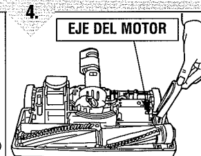
Diagrama 4 Saque la banda rota y reemplácela con una nueva.
