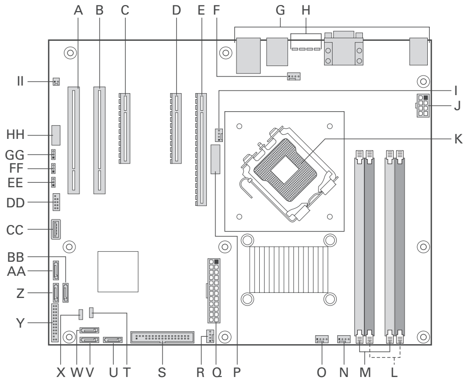
Figure 2. Emplacement des composants et des connecteurs sur la carte
