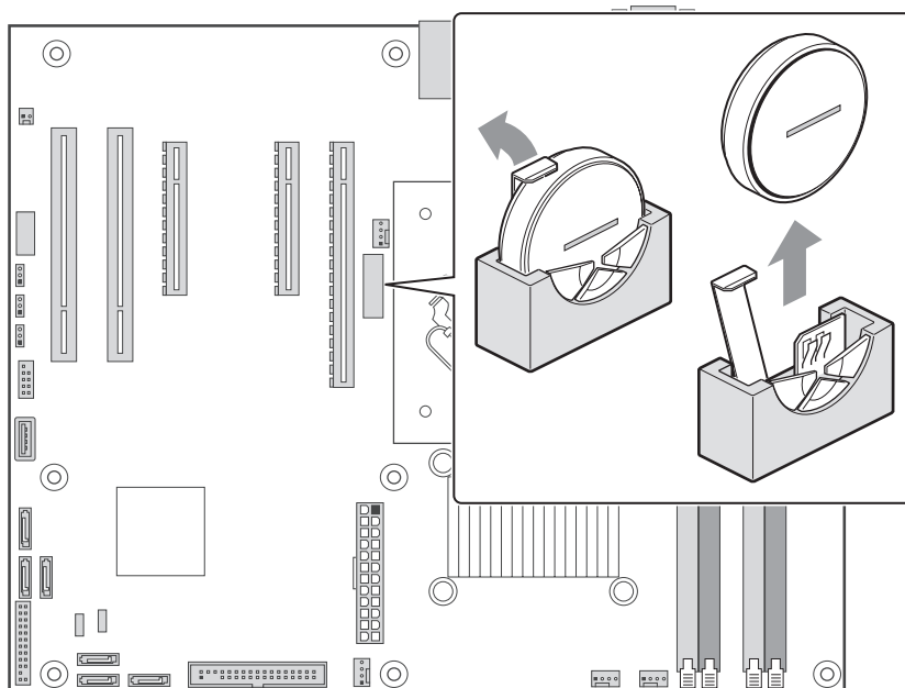
Figure 6. Remplacement de la pile
