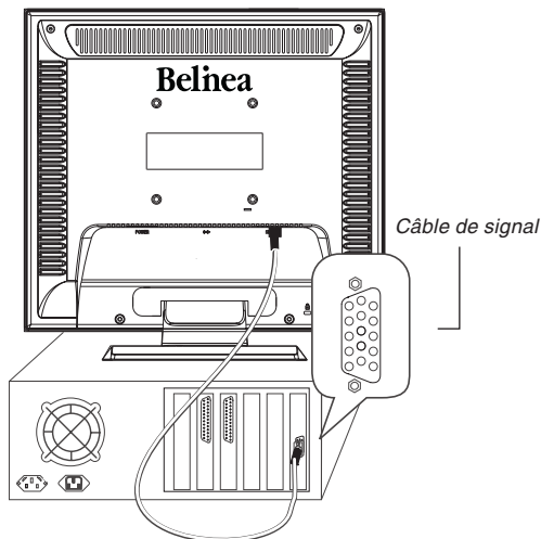
Figure 2. Raccordement du moniteur au PC
