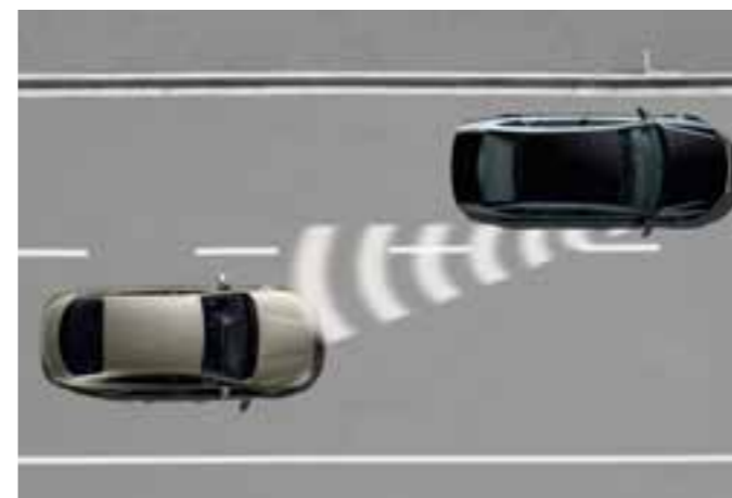
Le système d'assistance au changement de trajectoire "Side Assist plus", en option, vous aide à changer de file. Un signal visuel s'affiche sur le rétroviseur extérieur et vous avertit de la présence d'un véhicule dans "l'angle mort". Vous pouvez utiliser cette fonction dès que vous atteignez une vitesse de 30 km/h.
