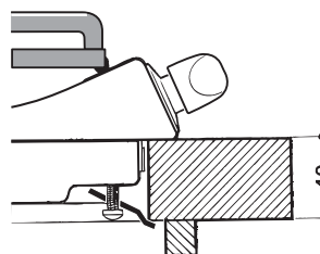
Position du crochet pour plan H=40mm
