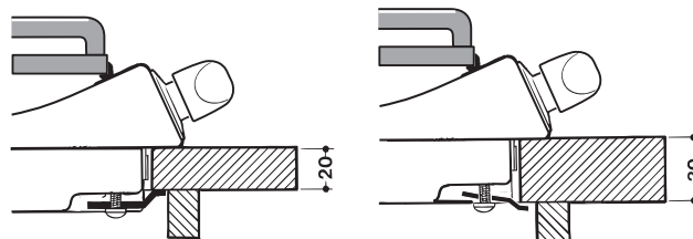
Position du crochet pour plan H=20mm
