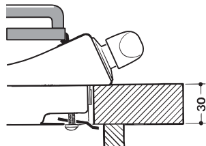
Posición del gancho para superficies H=30mm
