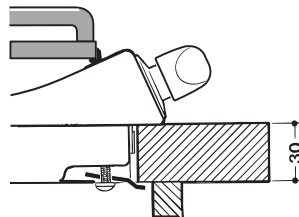
Posição do gancho para H=30mm
