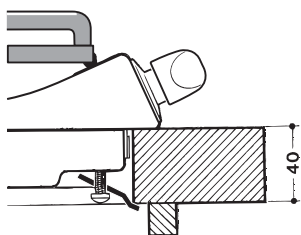
Posición del gancho para superficies H=40mm
