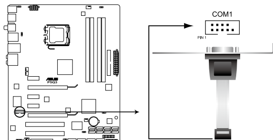
Connecteur du port série (COM1) de la P5Q3
