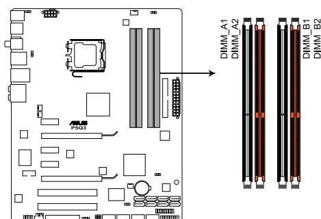
Sockets DIMM DDR2 de la P5Q3
