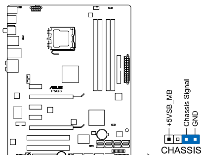
Connecteur du détecteur d'intrusion châssis de la P5Q3
