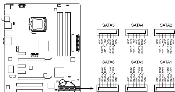
Connecteurs SATA de la P5Q3
