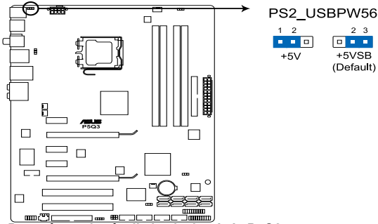
Paramètres de réveil via clavier de la P5Q3
