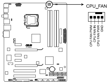
Connecteur CPU_FAN de la P5Q3
