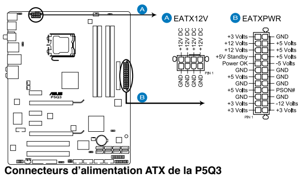
Connecteurs d'alimentation ATX de la P5Q3
