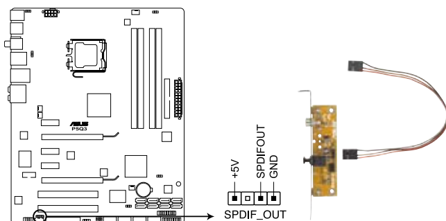
Connecteur audio numérique de la P5Q3
