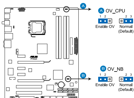
Paramètres de survoltage du CPU/Northbridge de la P5Q3
