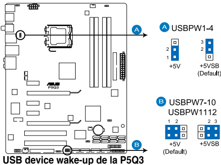
USB device wake-up de la P5Q3
