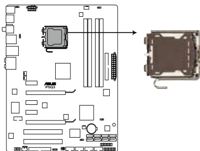
Socket 775 du CPU de la P5Q3
