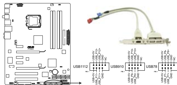
Connecteurs USB 2.0 de la P5Q3
