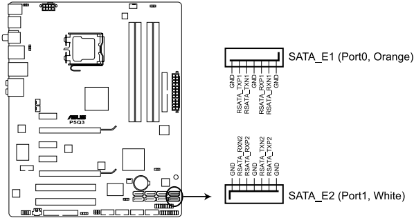
Connecteurs SATA (JMicron*) de la P5Q3
