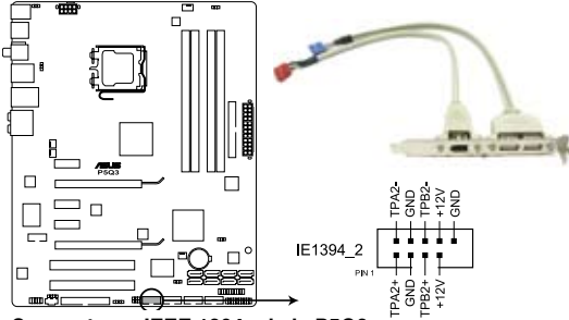
Connecteurs IEEE 1394a de la P5Q3
