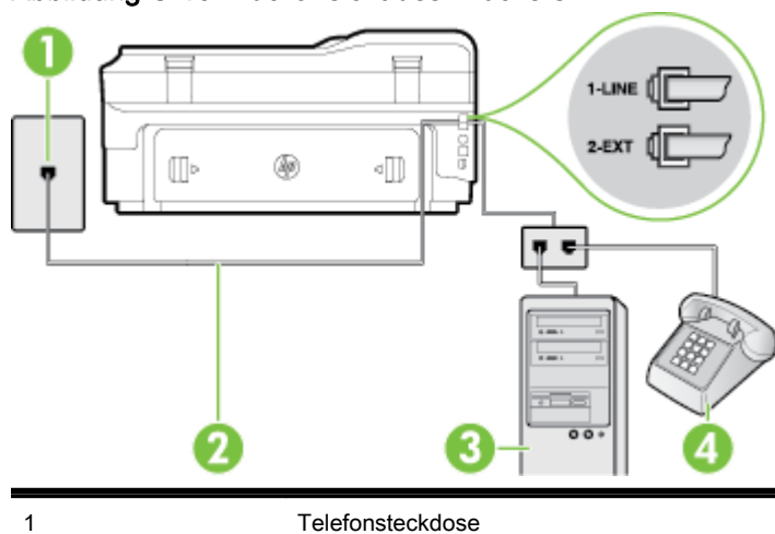
Abbildung C-16 Rückansicht des Druckers
