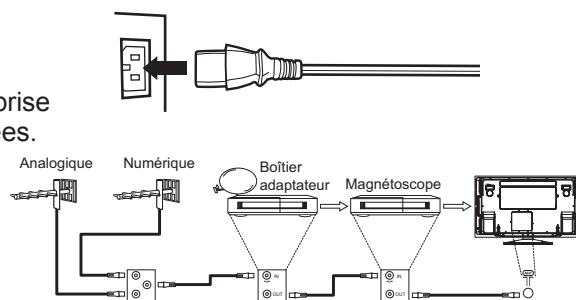
[Exemple: Connexion de l'antenne à travers un boîtier adaptateur et d'une magnétoscope]
