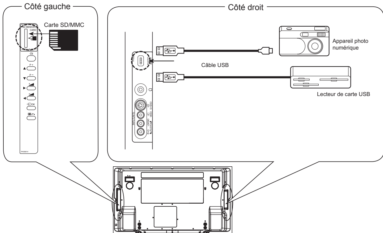
Panneau arrière (côté gauche et côté droit)
