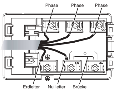
Dreiphasenanschluss 400
