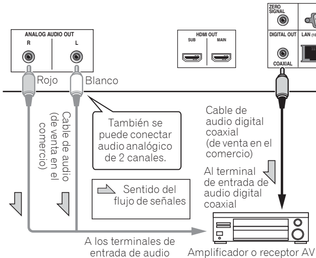
Panel posterior de BDP-LX58
