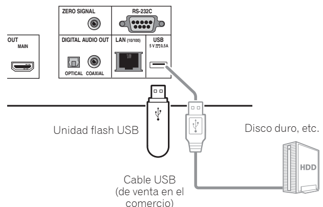
Panel posterior de BDP-LX88
