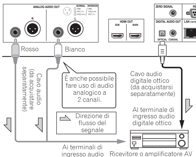
Pannello posteriore del BDP-LX88
