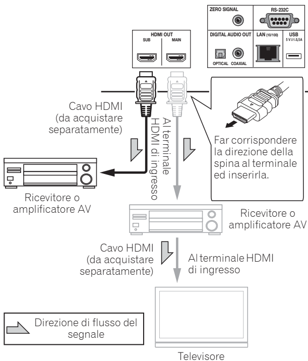
Pannello posteriore del BDP-LX88
