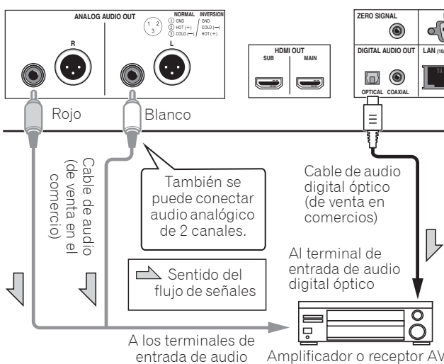
Panel posterior de BDP-LX88
