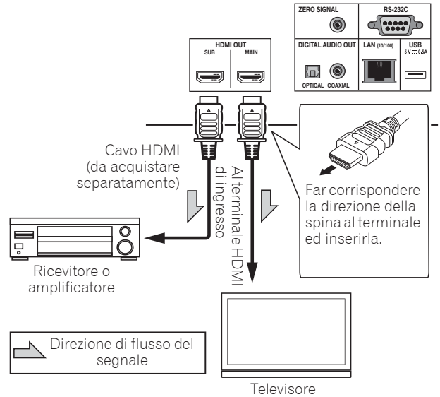
Pannello posteriore del BDP-LX88
