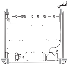
تركيب الخطافات بالنسبة للسطح الارتفاع=30 ملم
