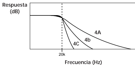
Comparación de las características de corte del filtro 4
