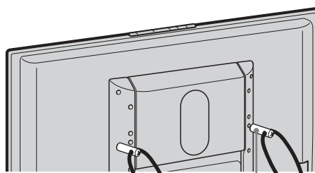
kabel (niet bijgeleverd) schroeven kantelbeveiliging (met gat)
