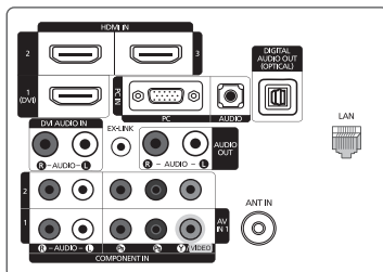
DÉTAILS DU PANNEAU DE PRISES
