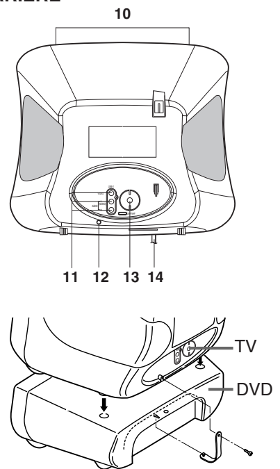
VUE ARRIERE
