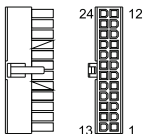
Connettore di alimentazione principale (24Pin)
