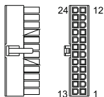
Conector principal de alimentación (24 pines)
