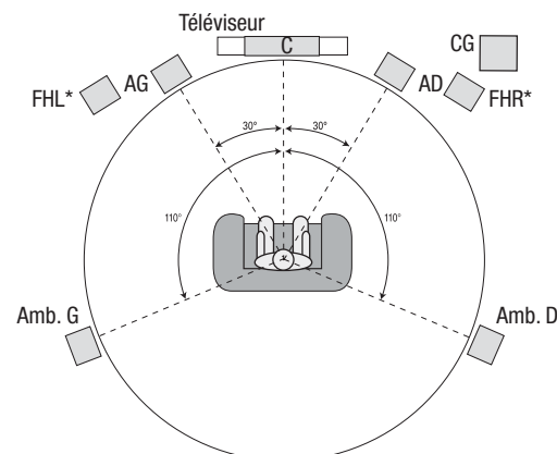
Positionnement des enceintes pour les systèmes canaux 7.1 (AVR 1710/AVR 171 uniquement) (Au milieu : avec des enceintes ambiophoniques arrière, En bas : avec des enceintes avant en hauteur)
