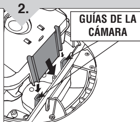
Diagrama 2 Vuelva a colocar la cámara de la bolsa con la bolsa en las guías de la cámara.
