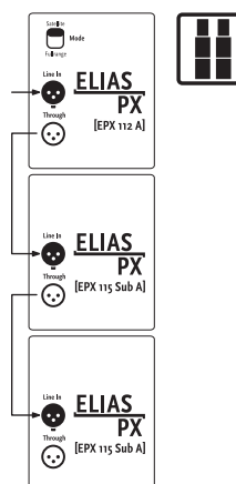
schéma de raccordement de l'Extension Set
