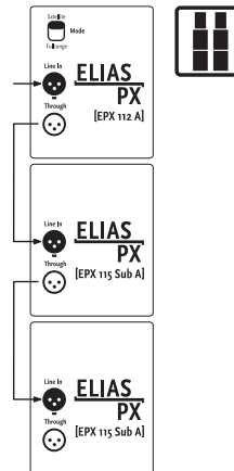
Esquema de conexión de Extension Set
