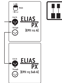
Anschluss-Schema Standard-System
