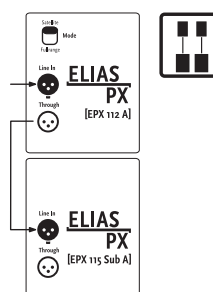
schéma de raccordement du système standard
