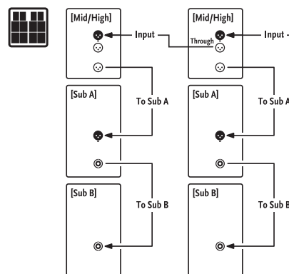
schéma de raccordement du système double
