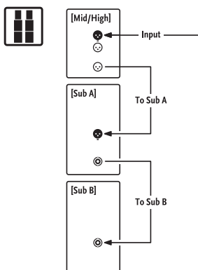
Anschluss-Schema Standard System
