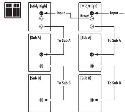
Esquema de conexión del sistema doble
