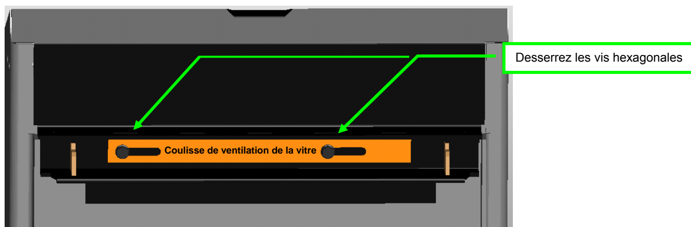
Amenez la coulisse sur la position souhaitée. Resserrez les vis hexagonales
