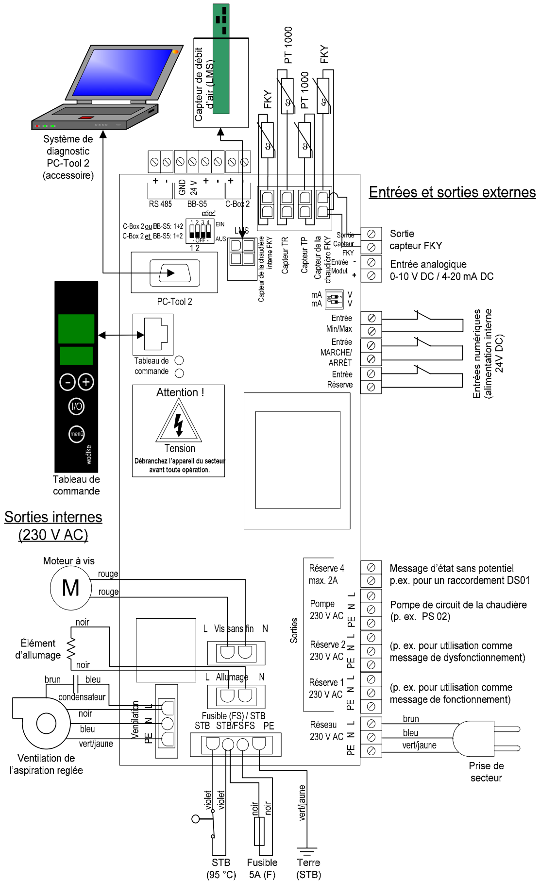
Plan de câblage et schéma de raccordement à la carte-mère principale
