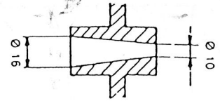
Réf. 010539 - Crépissage fin ou grosse tyrolienne
