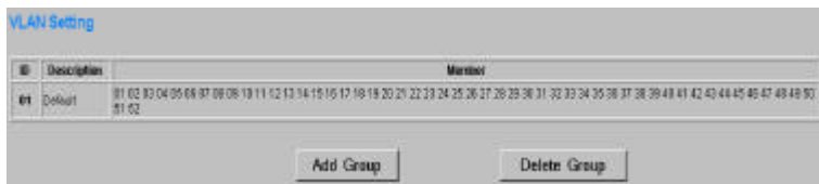
Figure 19. Paramètres des groupes de VLAN
