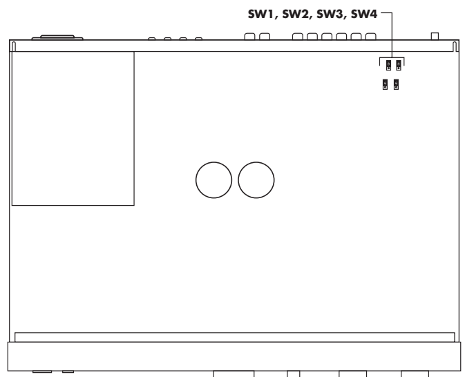
Figure 2: Phono/Line Input Jumpers Cavaliers de l'entrée Phono/Ligne Jumper für PHONO/LINE-Eingang Jumper Ingresso Linea/Phono Puentes de la Entrada Fono/Linea Doorverbindingstukjes voor p.u./lijn niveau aanpassing Omkopplare för skivspelar-/linjeingång Переключки для выбора режимов фоно/линейный вход
