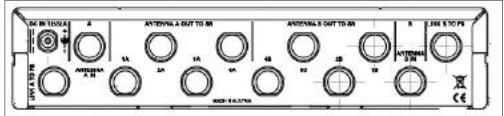
Fig. 2: Rückseite des PS 4000 W
