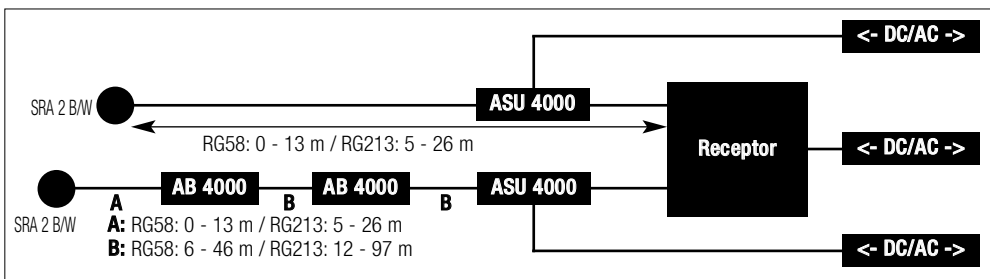
Fig. 7: Cablagem dum sistema monocal com antenas ativas e linhas de antenas de comprimentos diferentes
