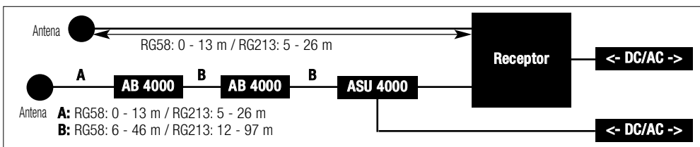
Fig. 6: Cablagem dum sistema monocal com antenas passivas e linhas de antenas de comprimentos diferentes
