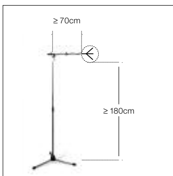
Fig. 3: Antenna montata su supporto da pavimento
