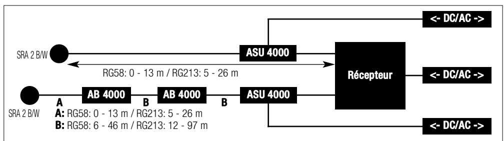
Fig. 7 : Câblage d'une installation monocanal avec antennes actives et différentes longueurs de câble.
