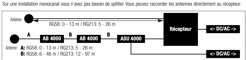
Fig. 6 : Câblage d'une installation monocanal avec antennes passives et différentes longueurs de câble
