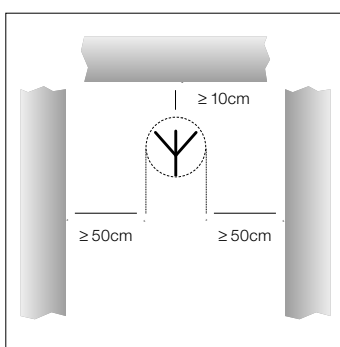
Fig. 4: Distanza minima da superfici piane
