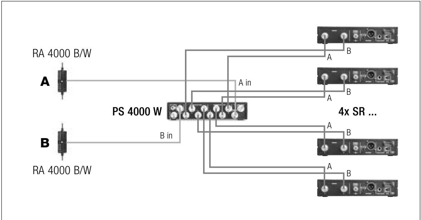
Fig. 10: Vierkanalanlage (Antennen, HF-Verbindungen) Four-channel system (antennas, RF connections) Système à quatre canaux (antennes, connections HF) Sistema con quattro canali (antenna, cablaggio RF) Sistema de cuatro canales (antenas, cableado de RF) Sistema de quatro canais (antenas, cablagem de RF)
