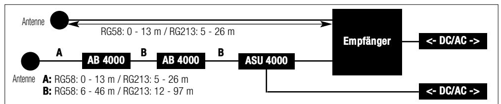
Fig. 6: Verkabelung einer Einkanalanlage mit passiven Antennen und unterschiedlich langen Antennenleitungen.
